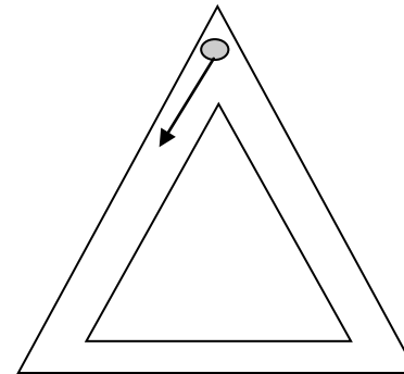
triangle équilatéral
