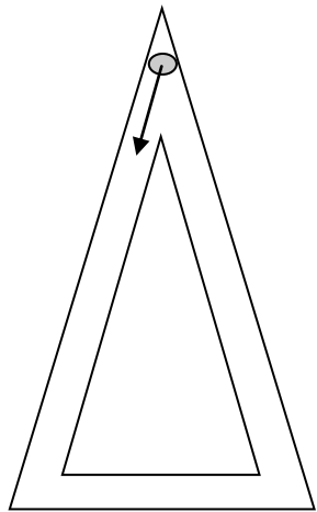
triangle isocèle
